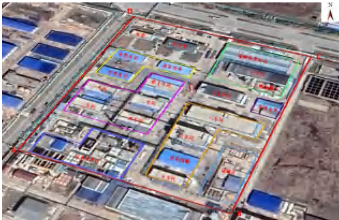
图4.2-1 厂区平面布置图
