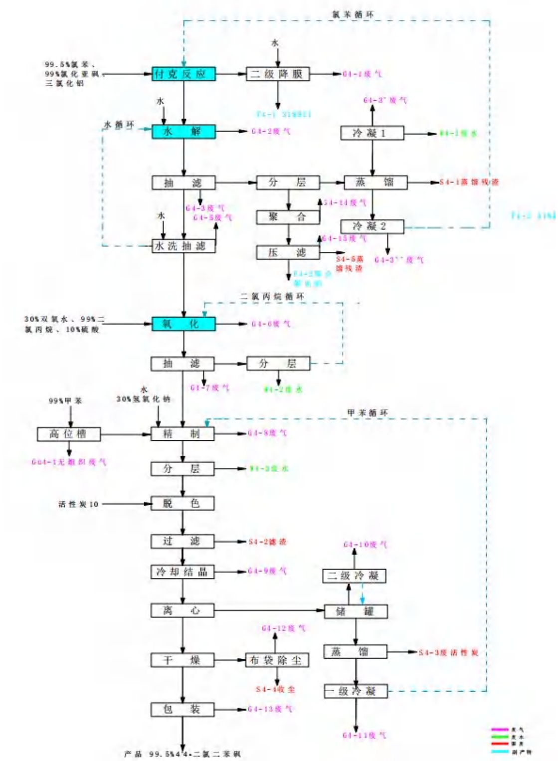
图 4-9 4,4'-二氯二苯砜生产工艺及产污节点图
